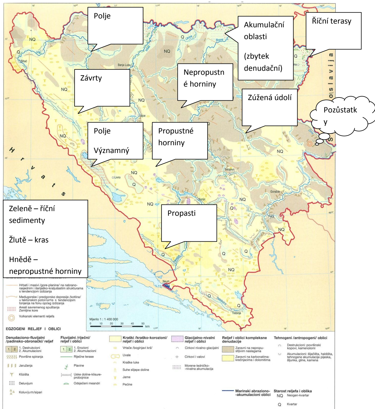
Obr. 3 Geomorfologie BaH
